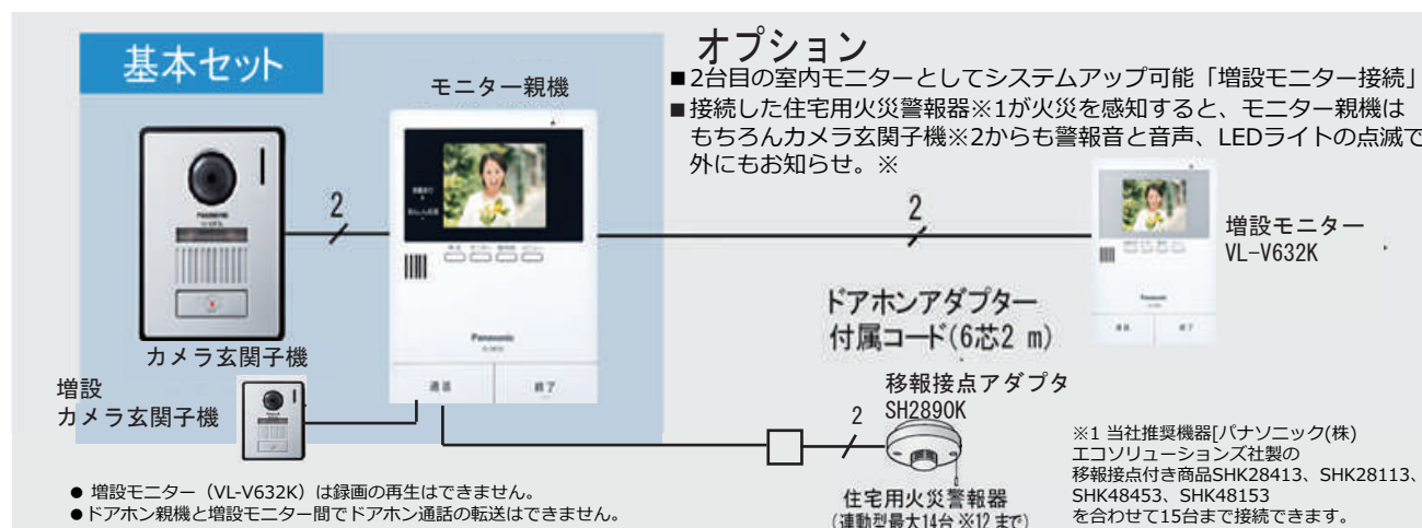
夜でもカラーで来訪者確認「LEDライト搭載」
